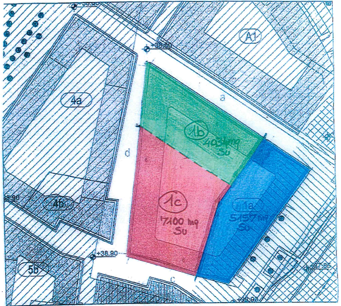
PLANIMETRIA 1:1000
